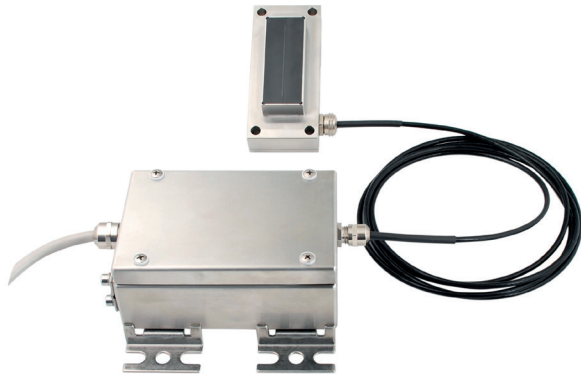
Meßumformer im Edelstahlgehäuse mit SONO- MIX Mini Standard Sonde
