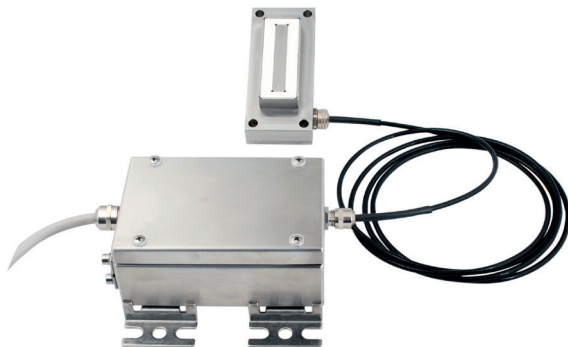
Meßumformer im Edelstahlgehäuse mit SONO- MIX Mini LD Sonde
