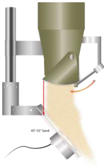
Sand: Einbauwinkel 45° bis 55°
